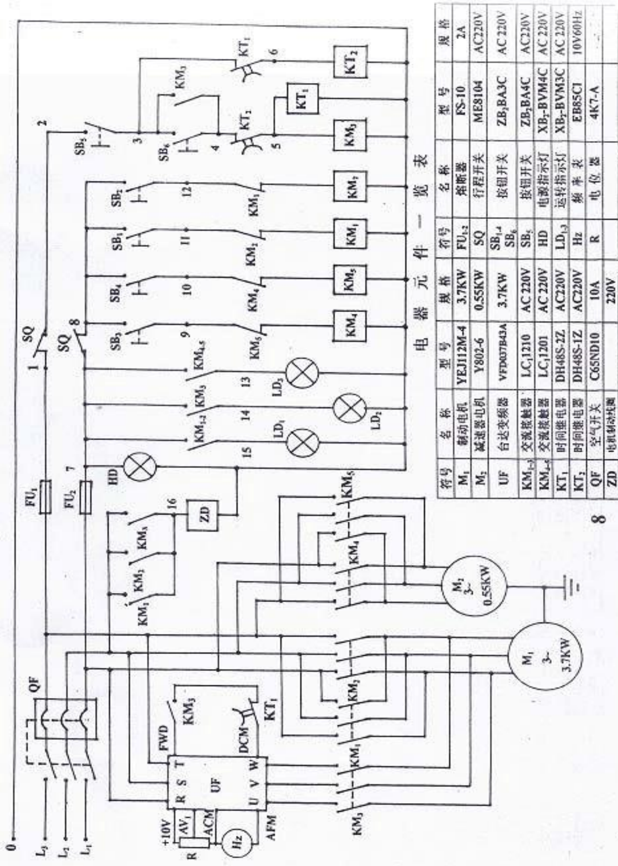
Рис. 3 Электрическая схема
